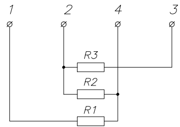
Схема электрическая принципиальная
